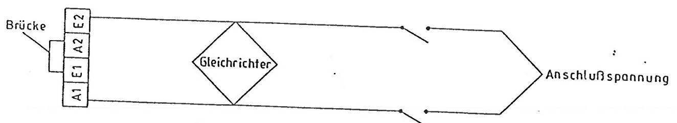
Abb.16: Anschlußpläne für Hub-(GH) und Spreizmagnete
