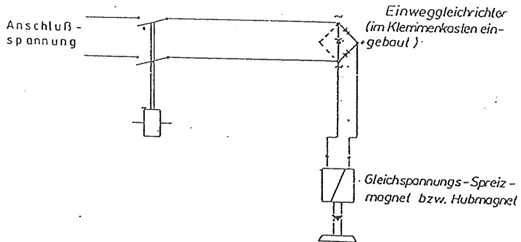
Schaltbild 2: (nur Hubmagnete)
