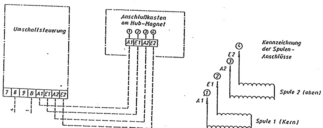
Schaltbild 2: (nur Hubmagnete)
